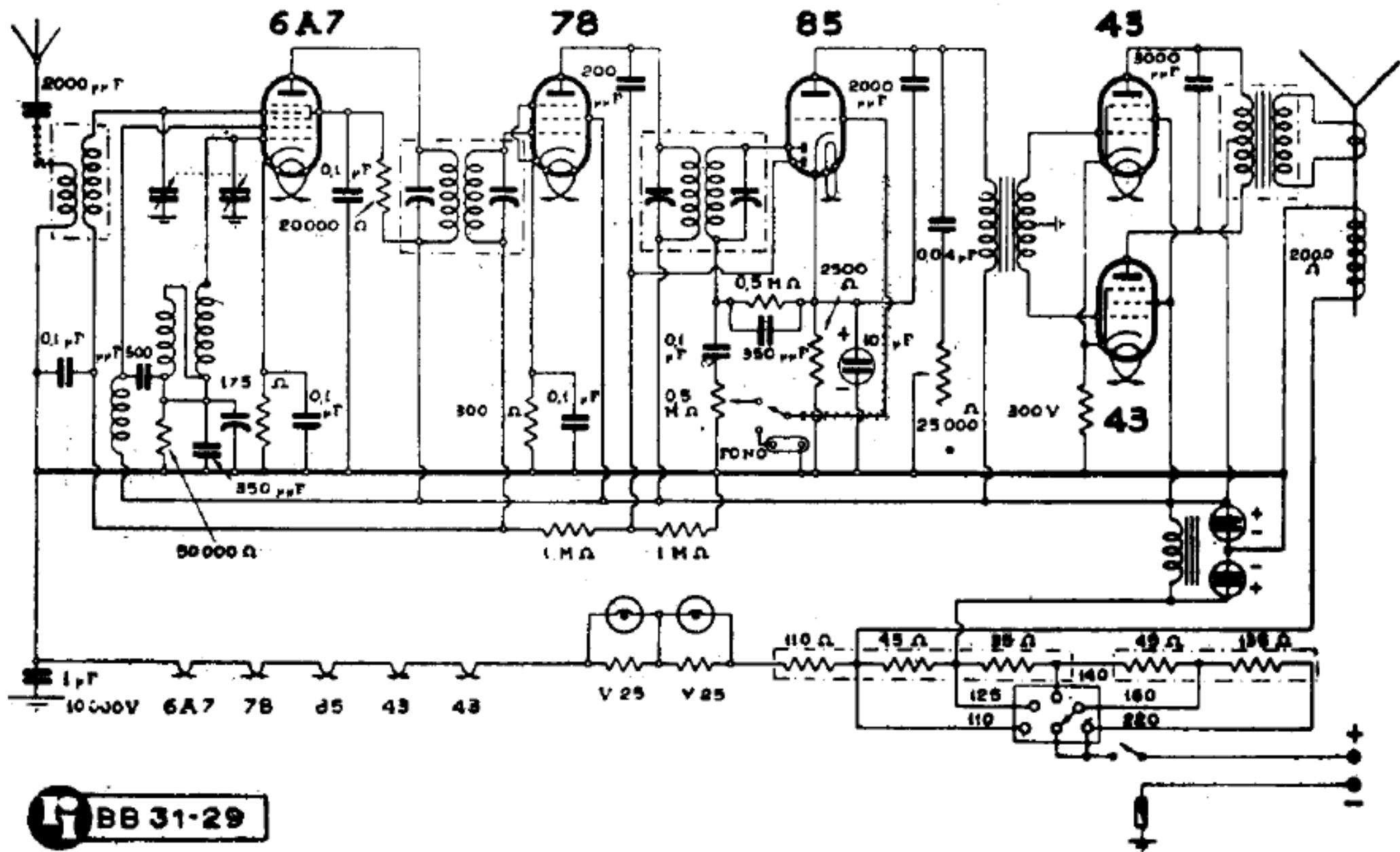
S.I.A.R.E. CROSLY - MOD. « 145 D »
